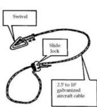
Fig. 31. Coyote snare
