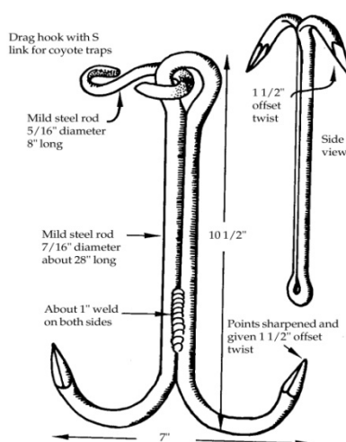
Fig. 30. Trapping drag
