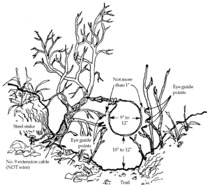
Fig. 37. Trail snare set
