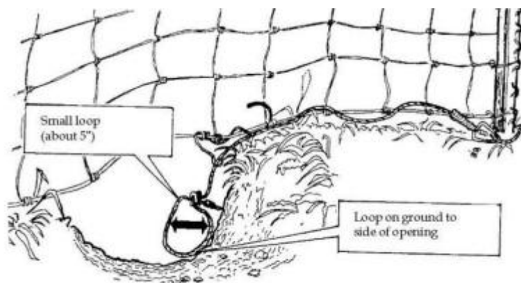
Fig. 36. Leg snare set
